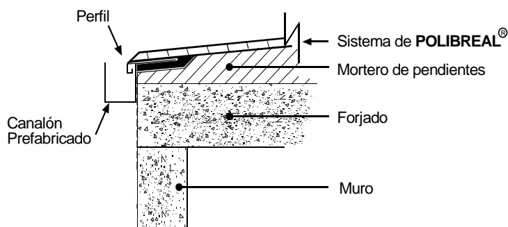
Figura 11- Entrega del sistema POLIBREAL® al borde extremo de un faldón con perfil metálico y canalón
