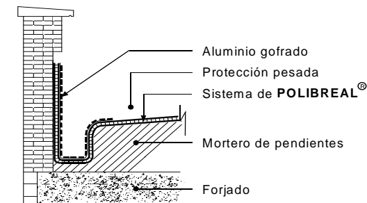
Figura 8- Canalón integrado en el borde del faldón
