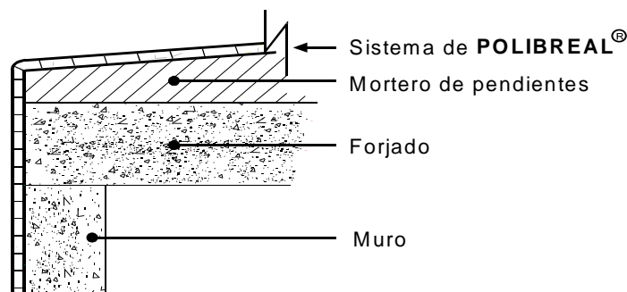
Figura 12- Entrega del sistema POLIBREAL® al borde extremo libre de un faldón
