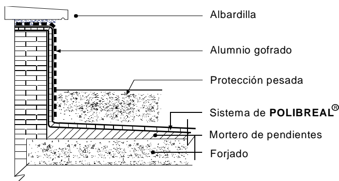
Figura 2- Entrega del sistema POLIBREAL autoprotectido a un paramento vertical
