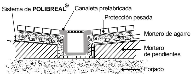
Figura 9- Canaleta prefabricada
