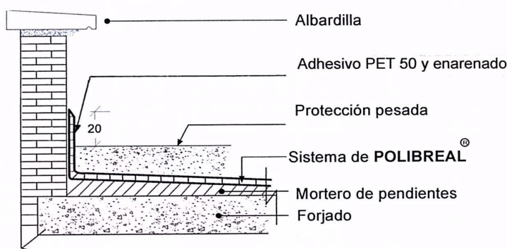
Figura 1- Entrega del sistema POLIBREAL a un paramento vertical.
