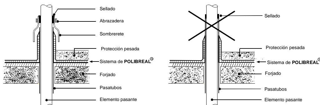
Figura 3- Pasa-tubos recto. Entrega del sistema POLIBREAL® con protección pesada. El hueco resultante entre pasa-tubos y elemento pasante, se cerrará mediante la colocación de un sombrerete.
