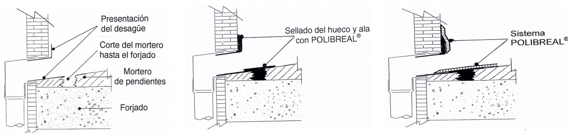
Figura 7- Sumidero horizontal
