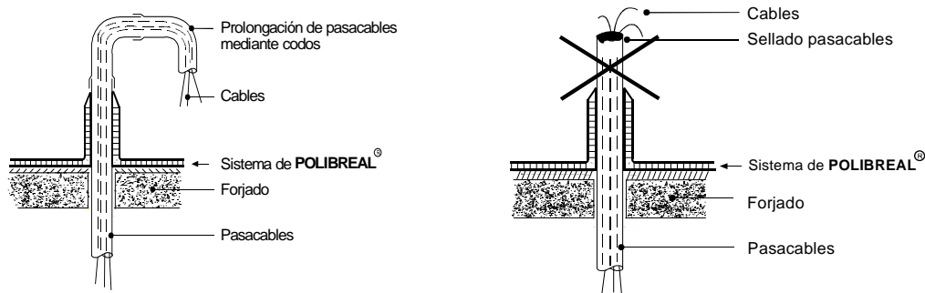
Figura 4- Pasa-cables curvado. Entrega del sistema POLIBREAL® con autoprotección metálica
