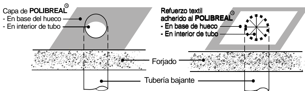
Figura 10- Bajante enrasada con el faldón
