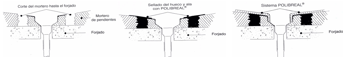
Figura 5- Sumidero vertical sobre formación de pendientes
