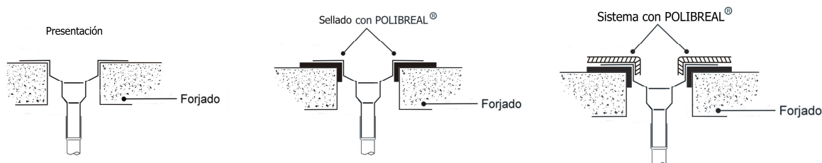
Figura 6- Sumidero vertical sobre forjado resistente
