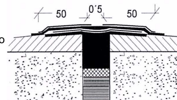
Figura 13- Tratamiento de junta paso a paso
